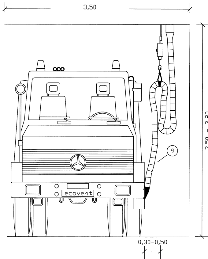
Frontansicht LS 10-D
