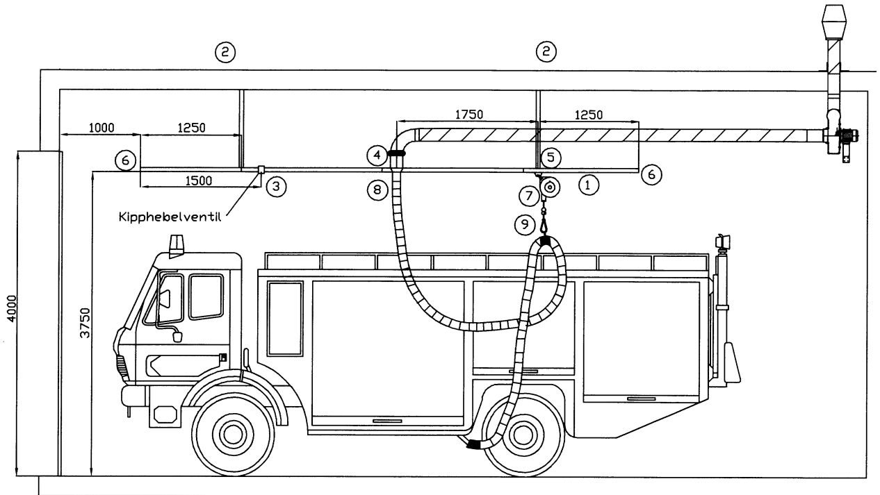
Seitenansicht LS 10-D
